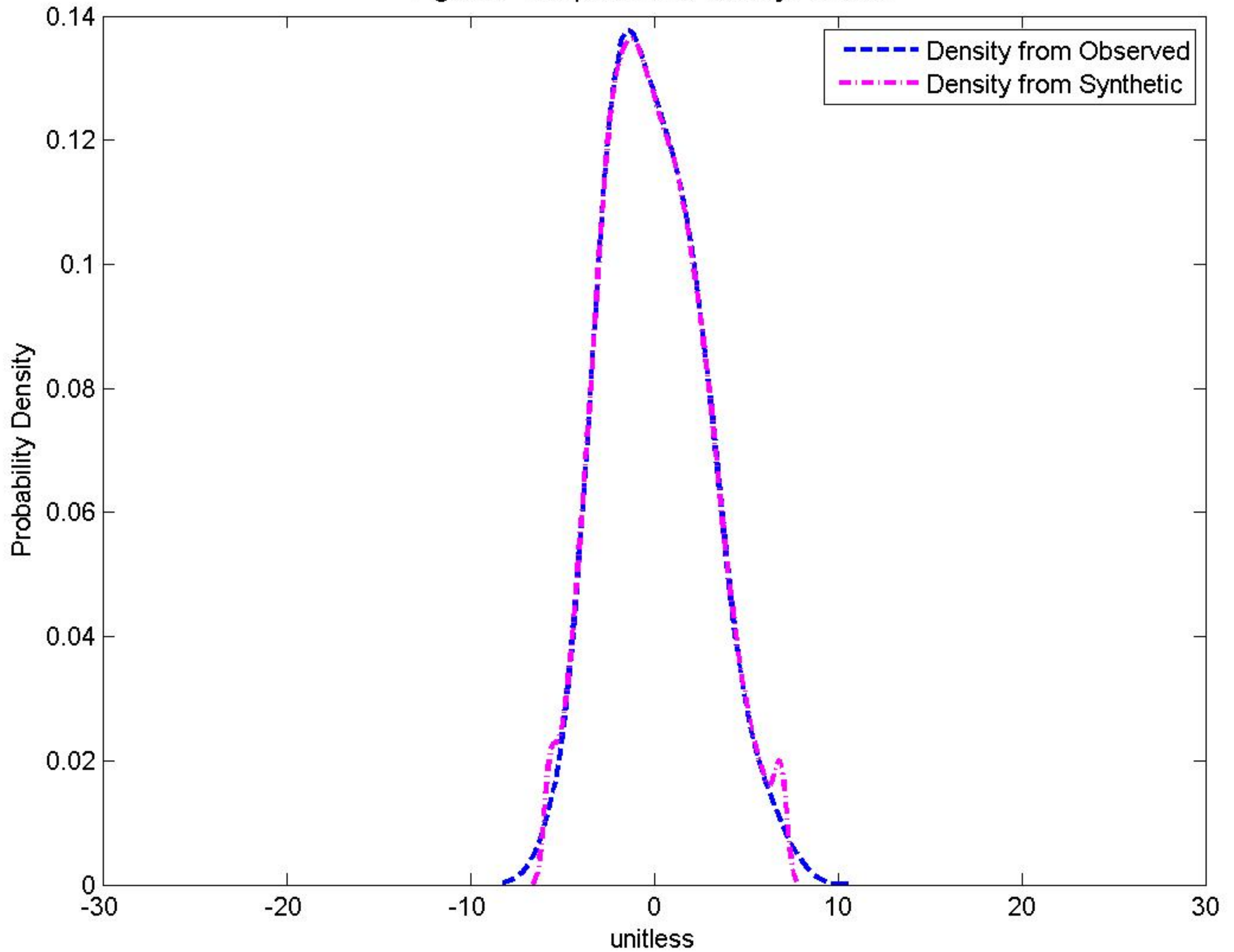
Fig.G13 - Nonparametric Density Function
