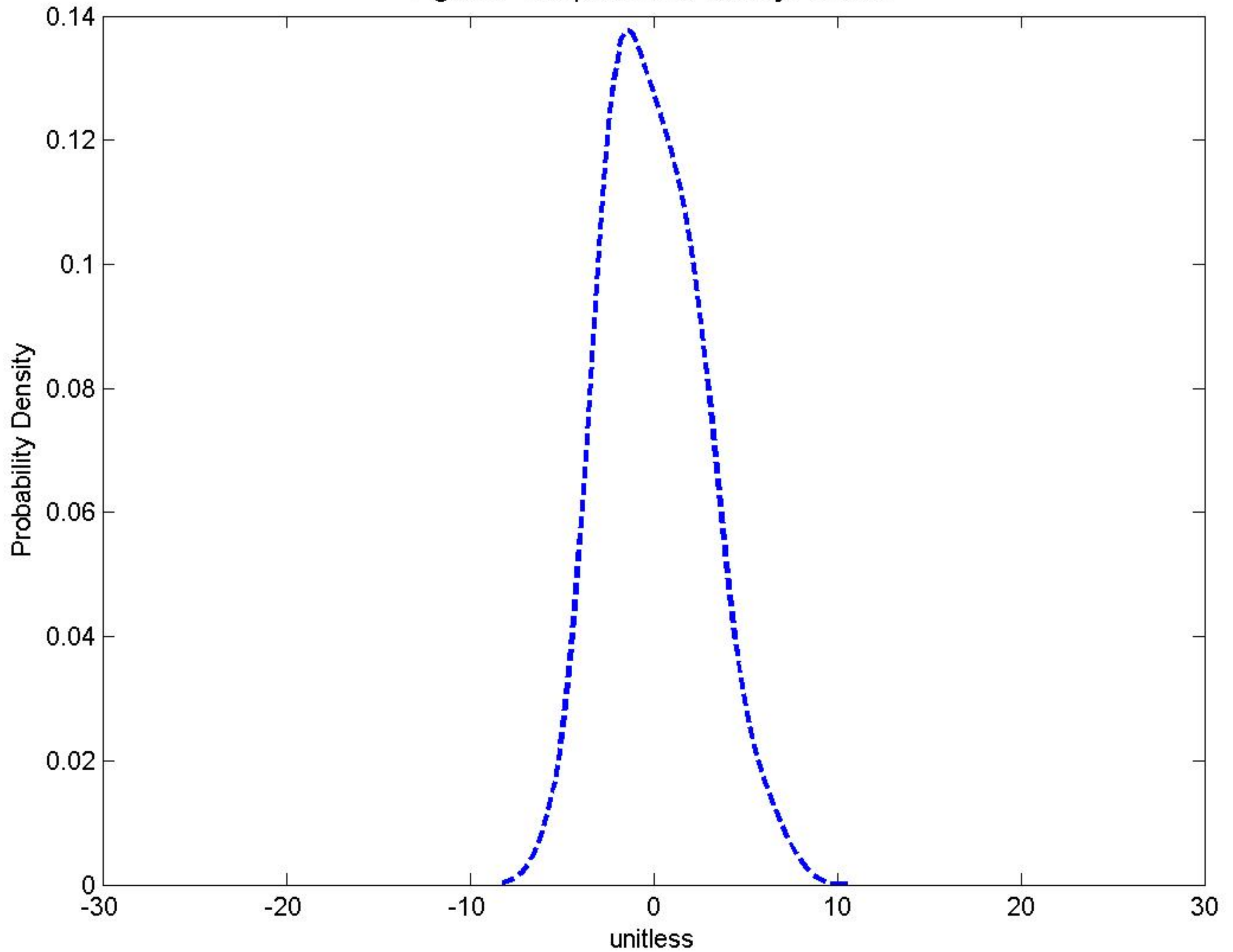
Fig.G10 - Nonparametric Density Function
