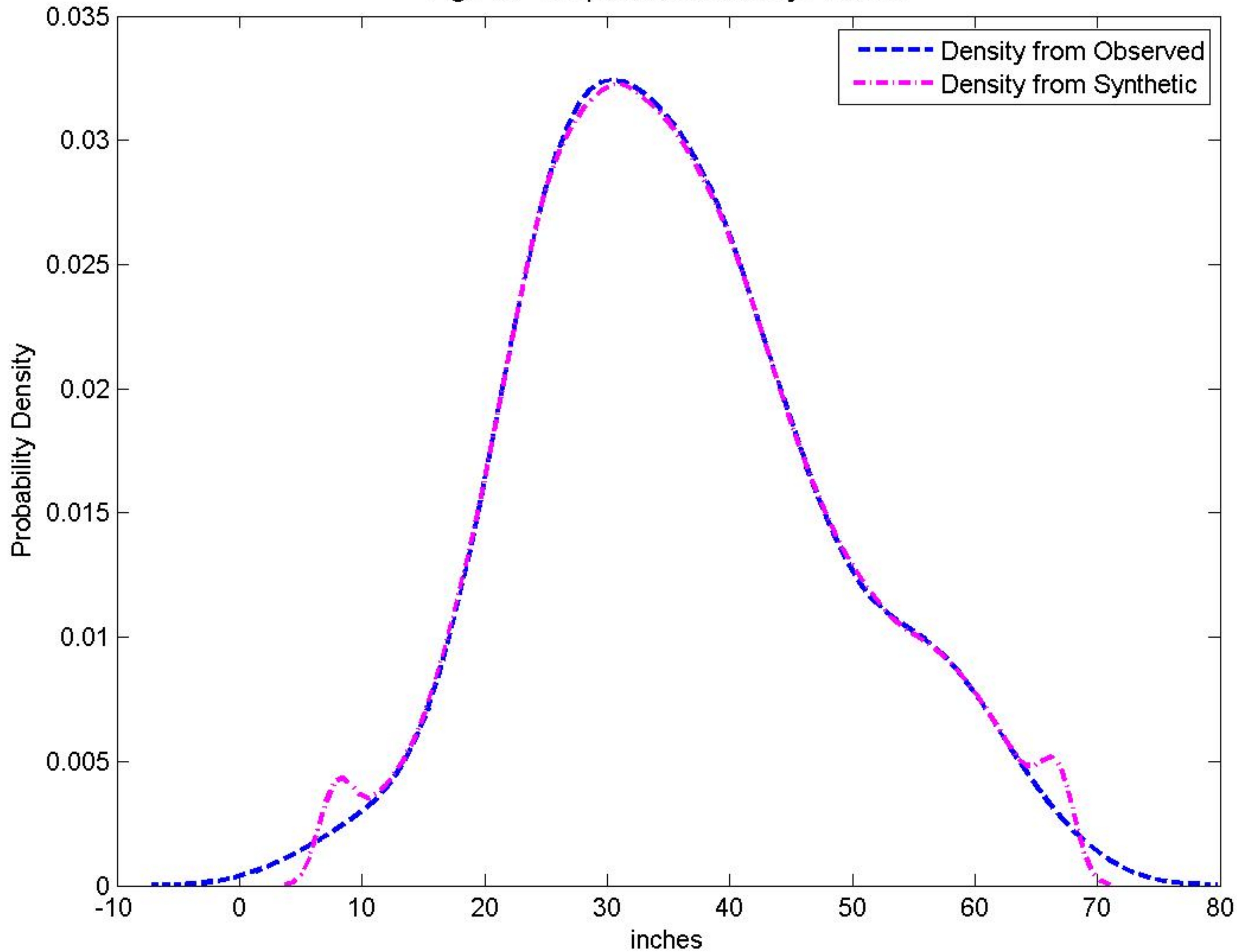
Fig.F13 - Nonparametric Density Function
