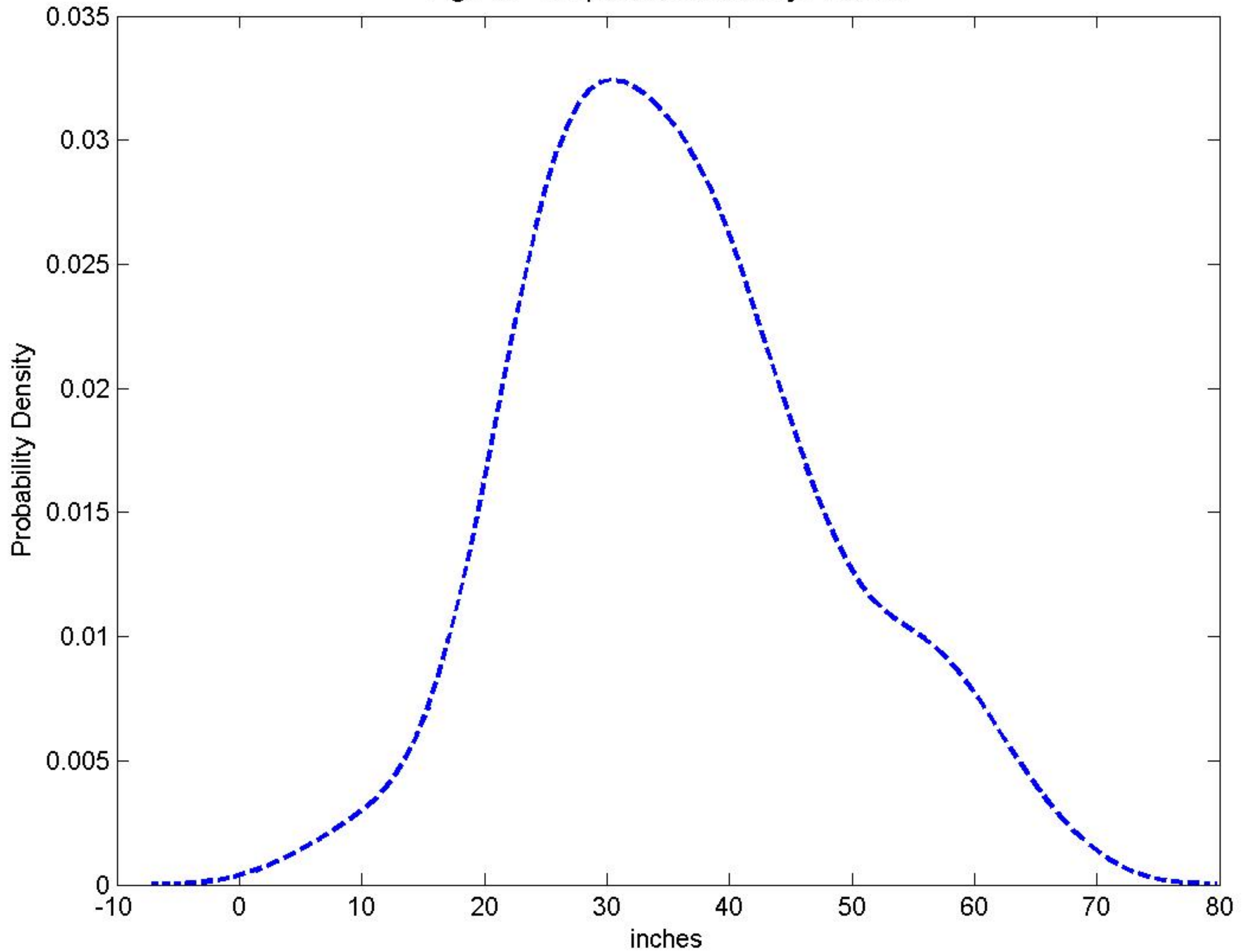
Fig.F10 - Nonparametric Density Function
