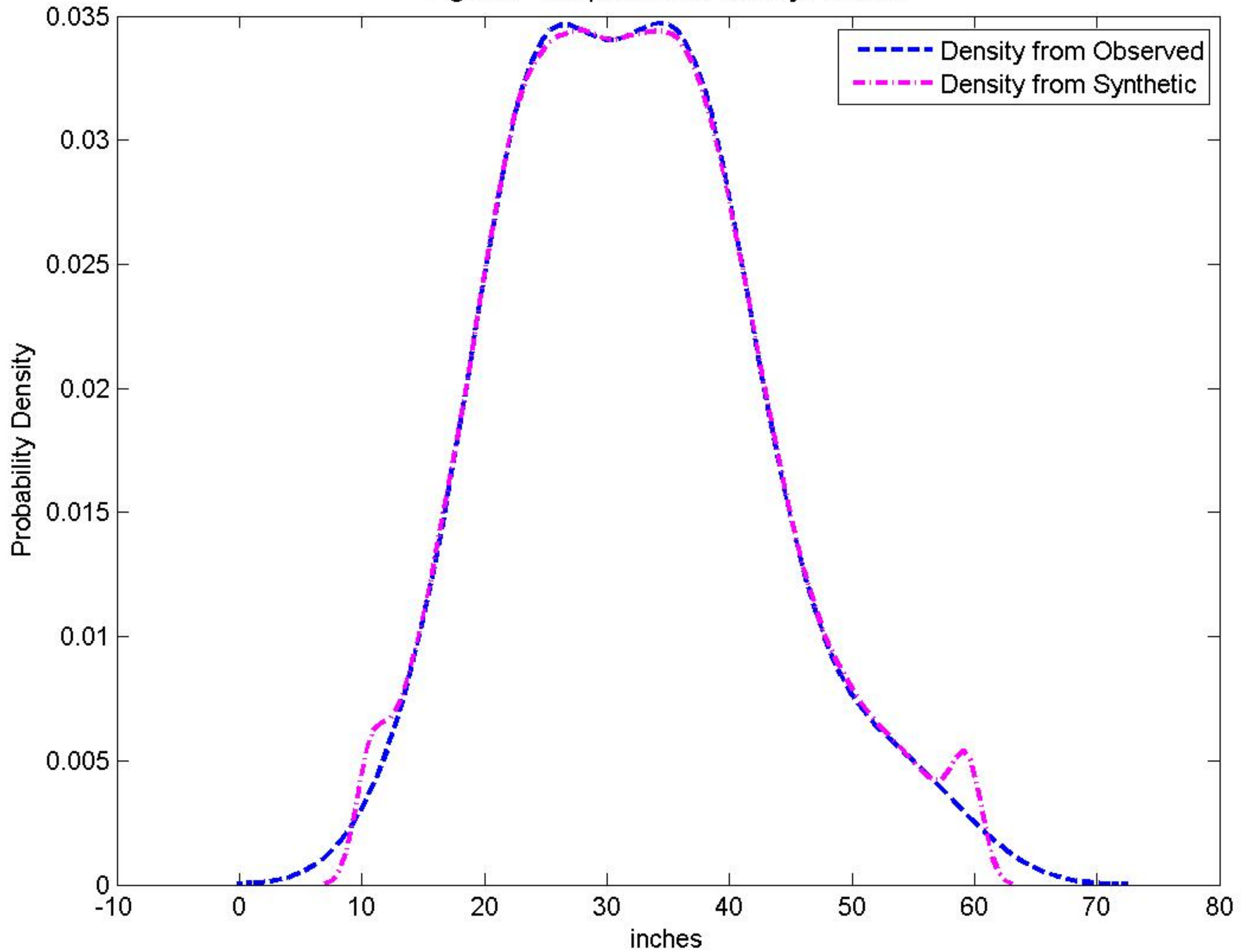
Fig.D13 - Nonparametric Density Function
