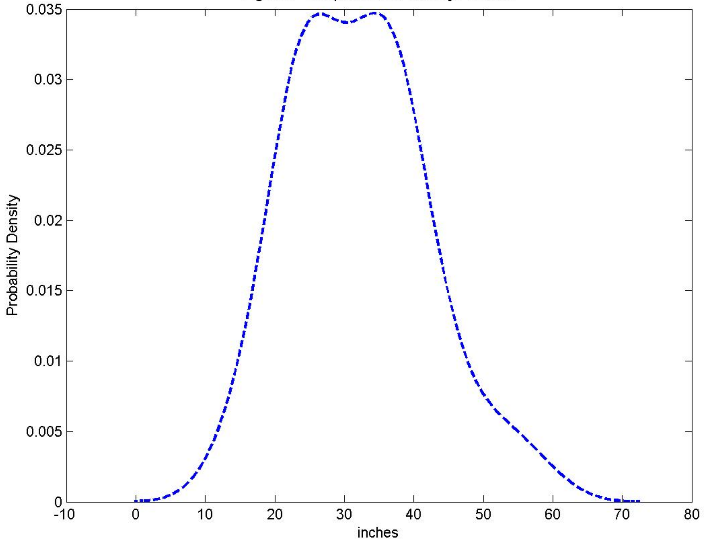
Fig.D10 - Nonparametric Density Function
