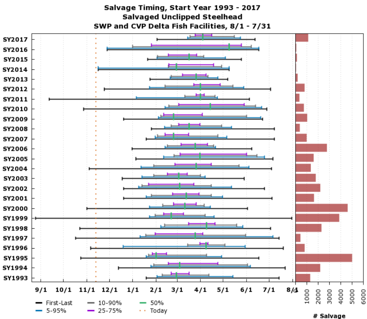
Figure 5.10-20. Sac PAS Salvage Unclipped Steelhead
